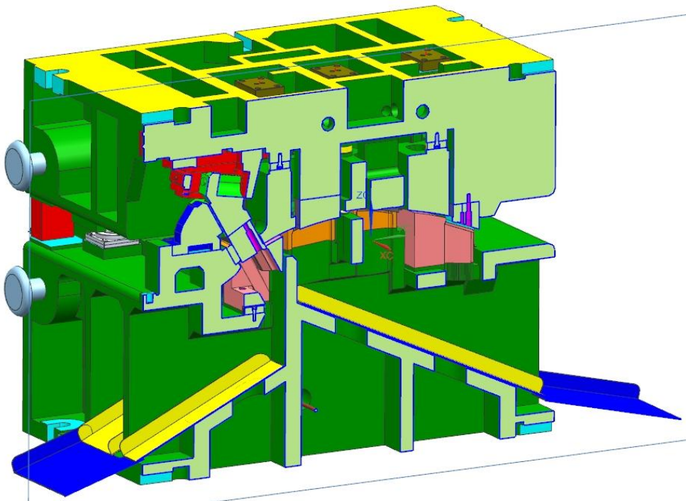
EX11-8889001618-822-左右前轮罩侧加强梁外板-OP30 模具---剖视图
