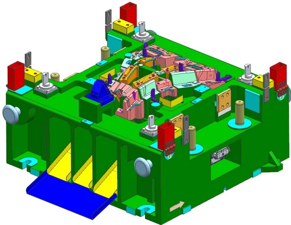
EX11-8889001618-822-左右前轮罩侧加强梁外板-OP30 模具---下模轴侧图
