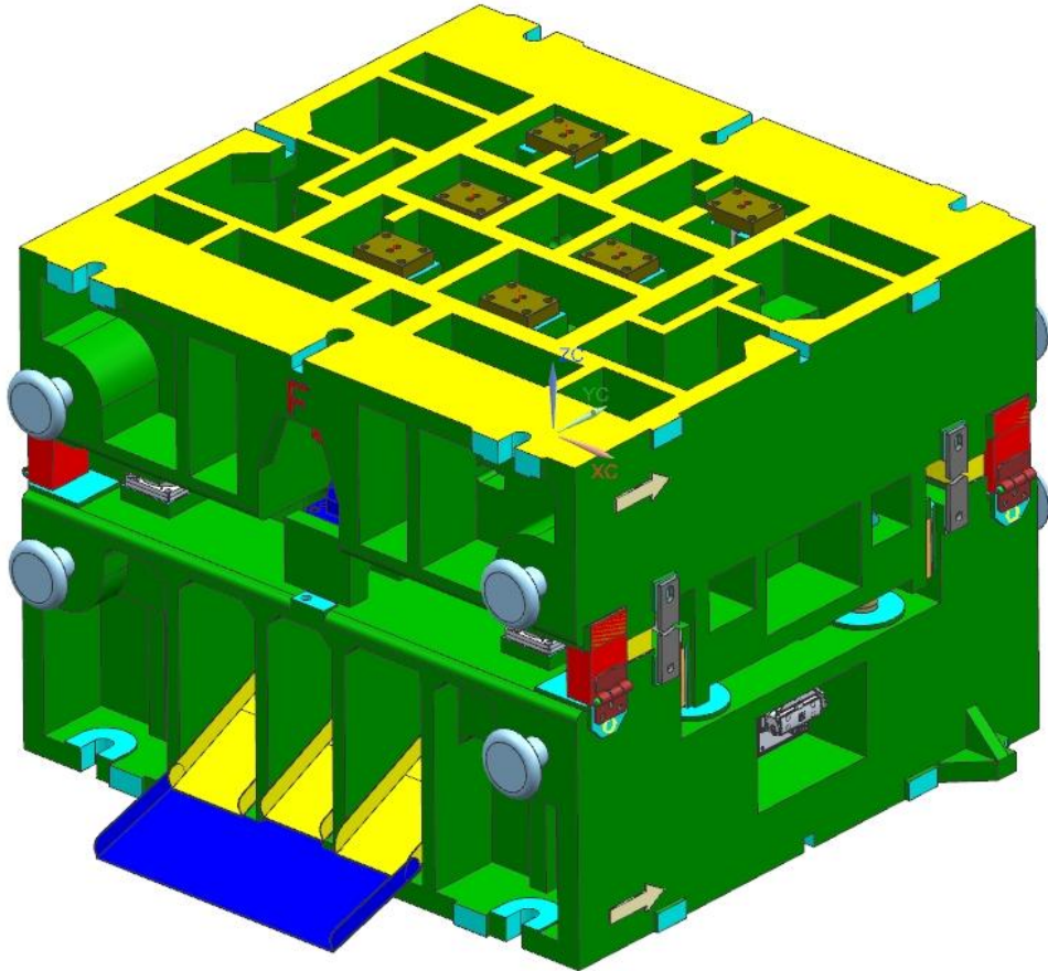
EX11-8889001618-822-左右前轮罩侧加强梁外板-OP30 模具---轴测图
