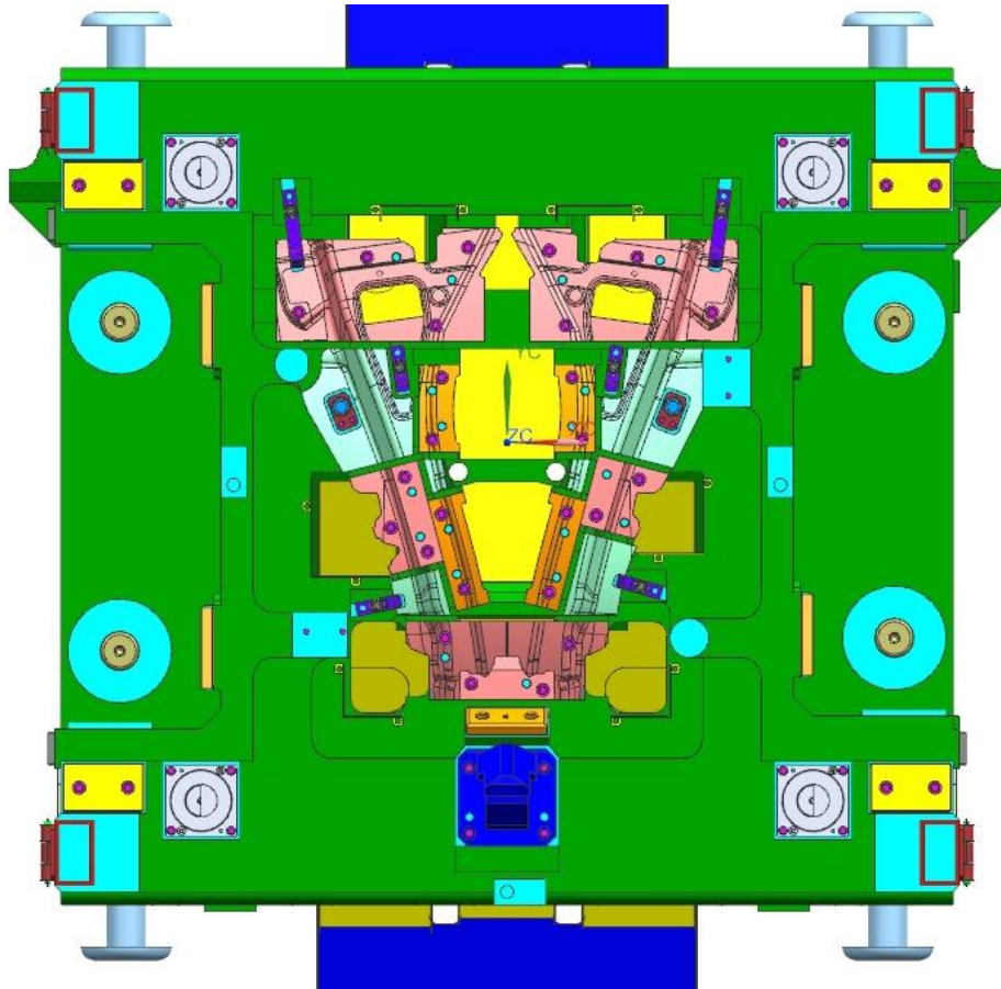
EX11-8889001618-822-左右前轮罩侧加强梁外板-OP30 模具---下模平面图
