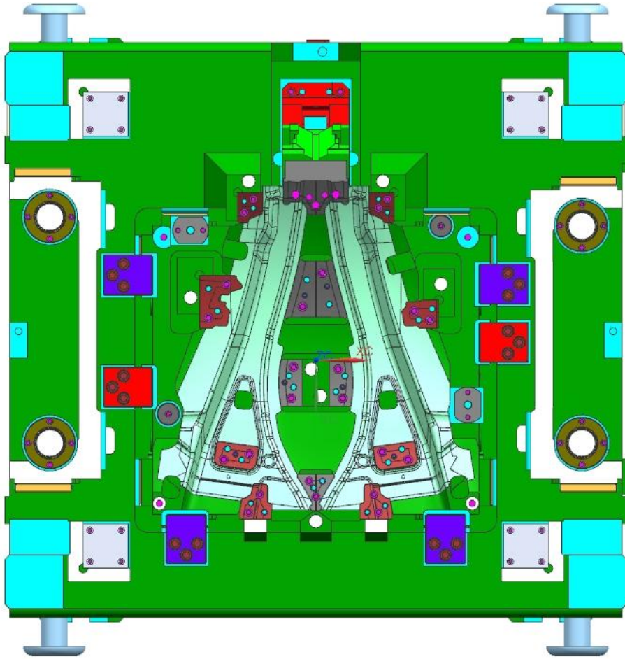
EX11-8889001618-822-左右前轮罩侧加强梁外板-OP30 模具---上模平面图
