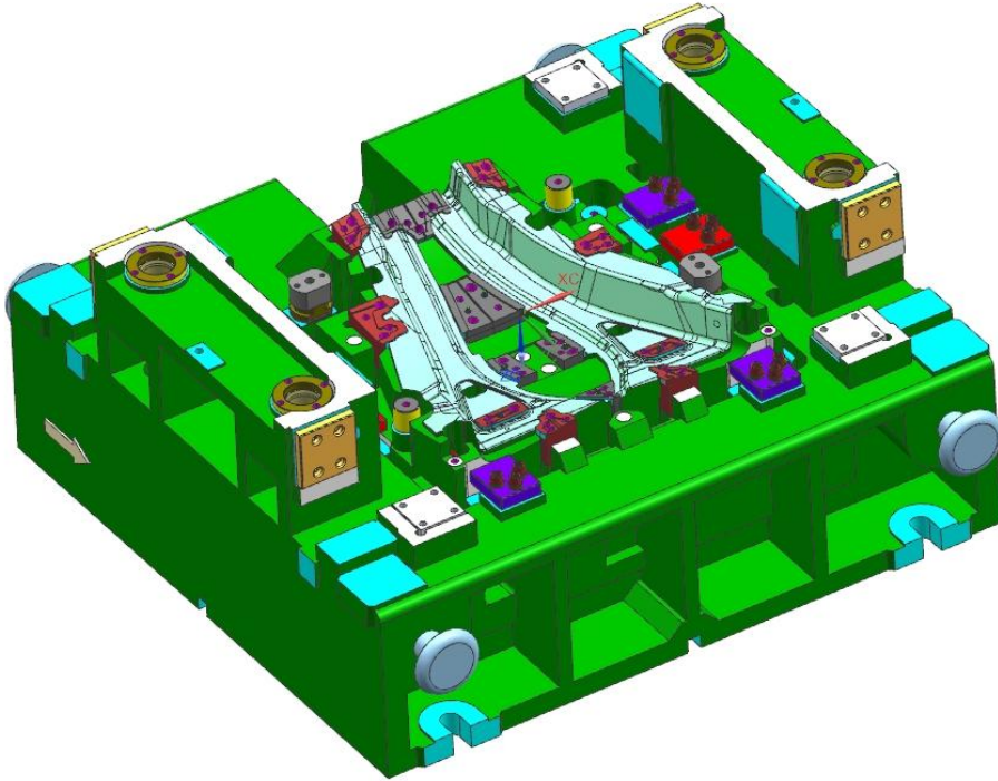
EX11-8889001618-822-左右前轮罩侧加强梁外板-OP30 模具---上模轴侧图
